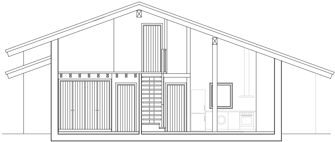
SECCION LONGITUDINAL
