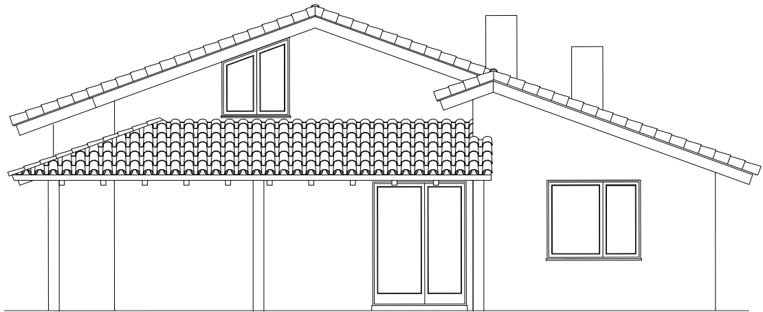
ALZADO LATERAL IZQUIERDO
